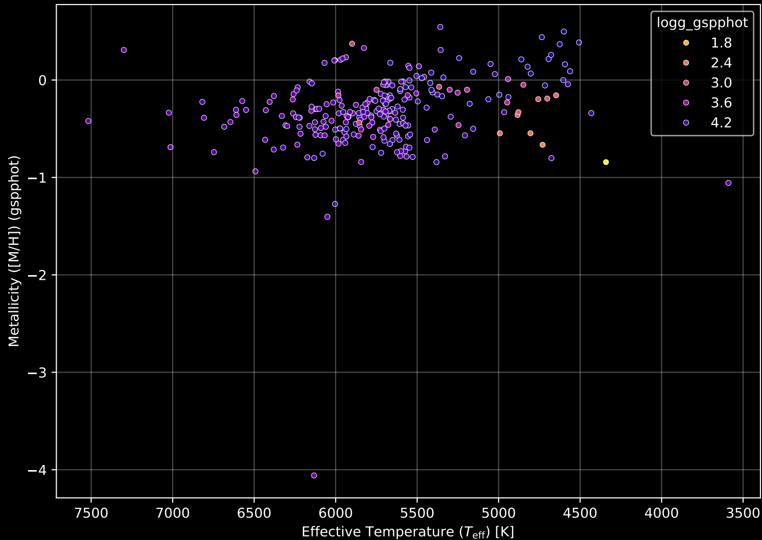
GALAH DR4 Field: [567] Stellar Population Parameters (n= 259)
