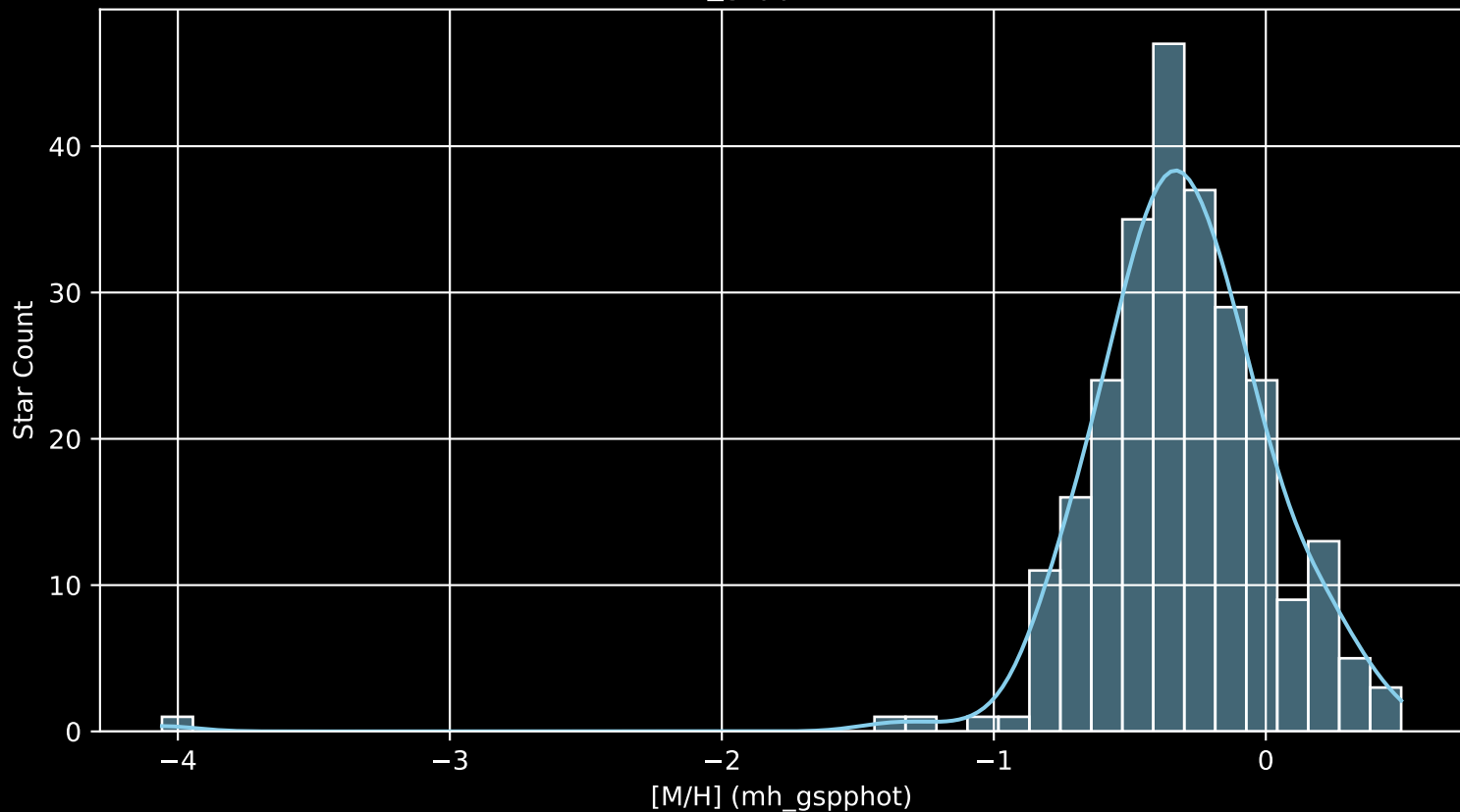
GALAH DR4 Field: [567] [M/H] (mh_gspphot) (n= 258)
