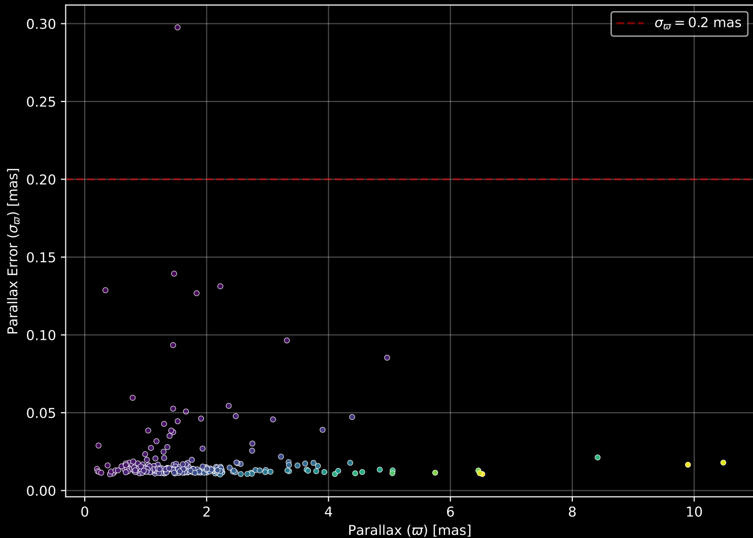
GALAH DR4 Field: [567] Parallax Quality (n= 259)
