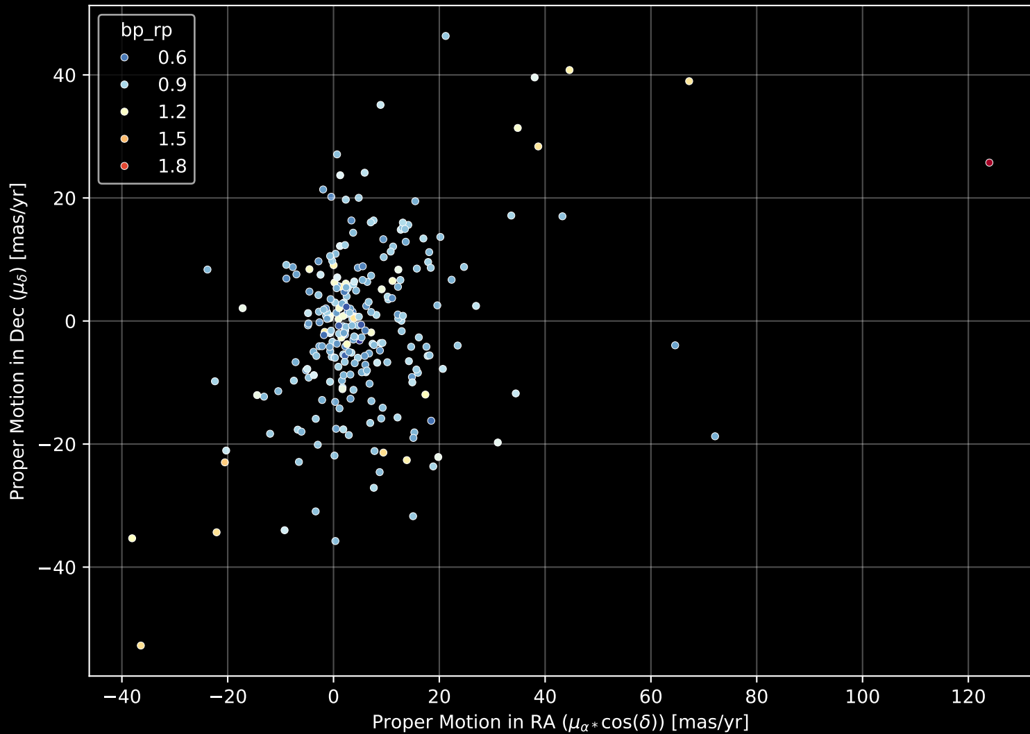
GALAH DR4 Field: [567] Proper Motion Diagram (n= 259)
